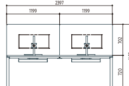
シングルモニターアーム 無段階で高さ調整/ 首振り角度調整が可能。 支柱高さ: 385mm VESA規格: 75×75/100×100 推奨モニターインチ: ~30インチまで 耐荷重: 10kg
